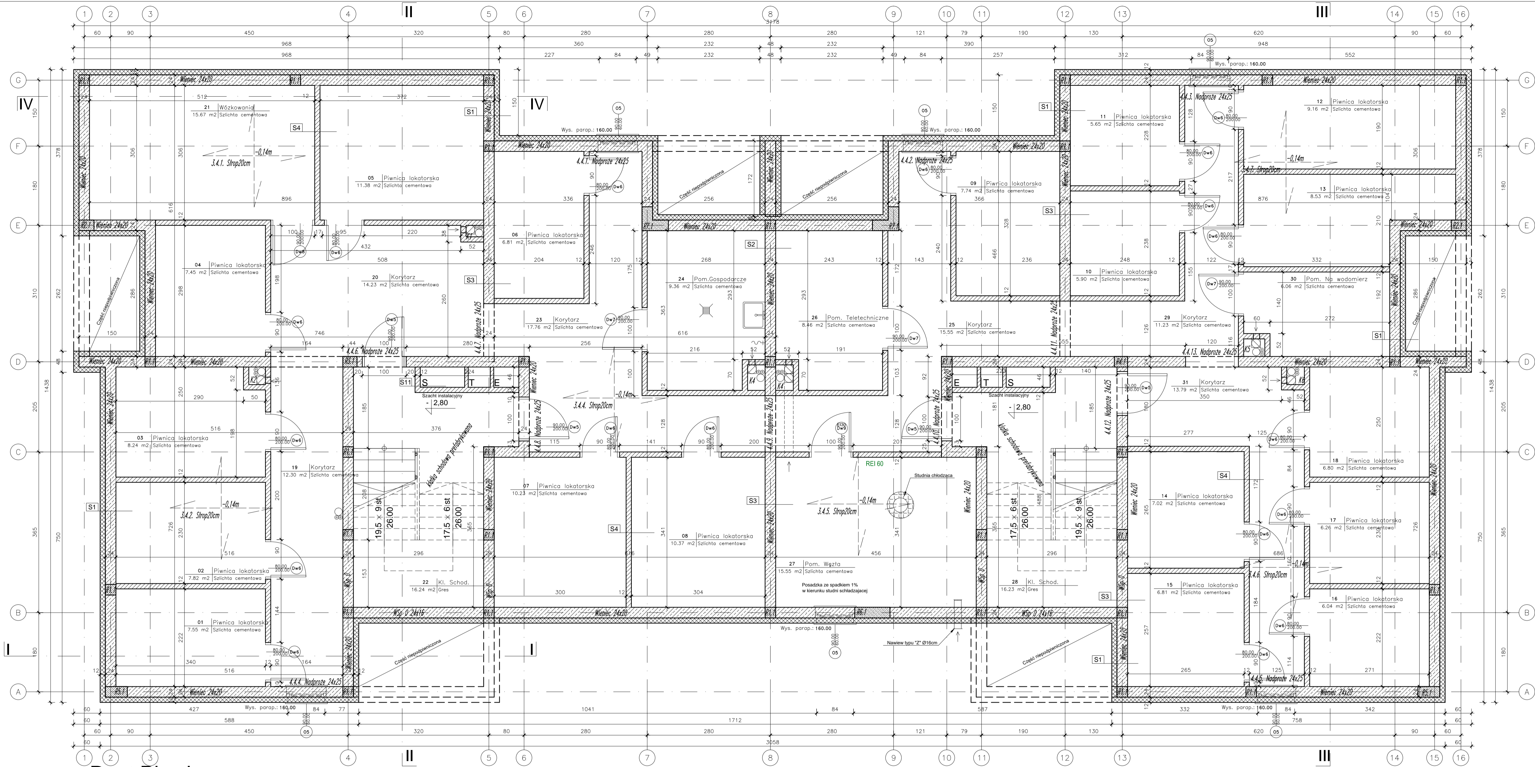
Rzut Piwnicy skala 1:50
